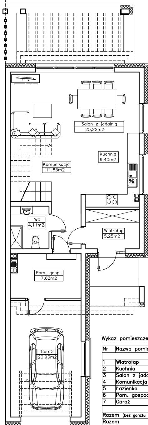
RZUT PRZYZIEMIA
